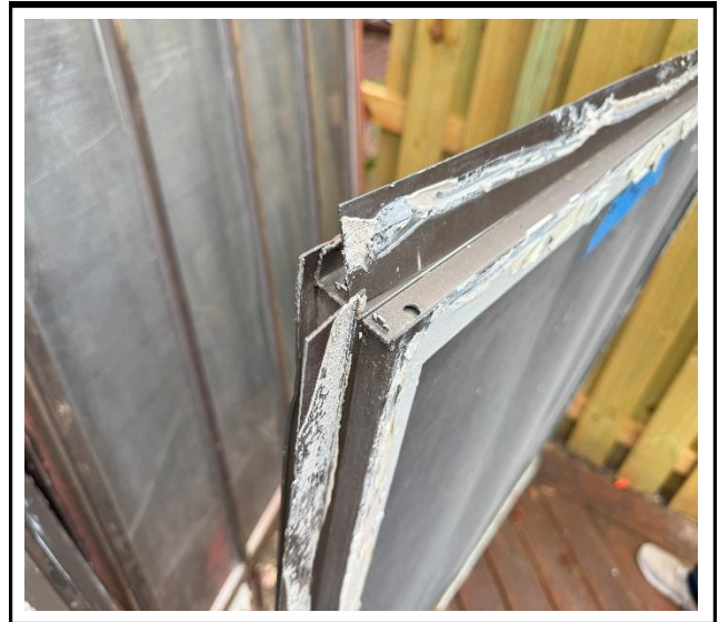
Photo 2 : Bad Frame
